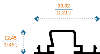
6022 TAPA BOLSA
