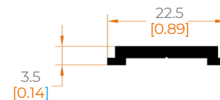
1506 PLETINA CREMONA
