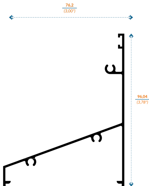
10467/6221 REPISÓN
