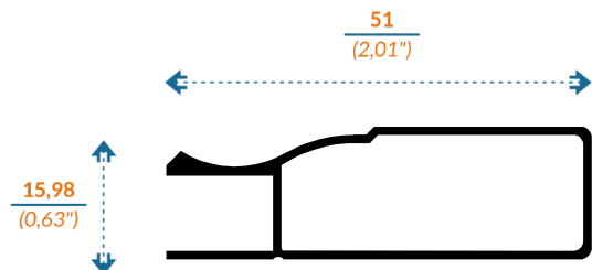
11173/17624 MARCO LUJO (1)
