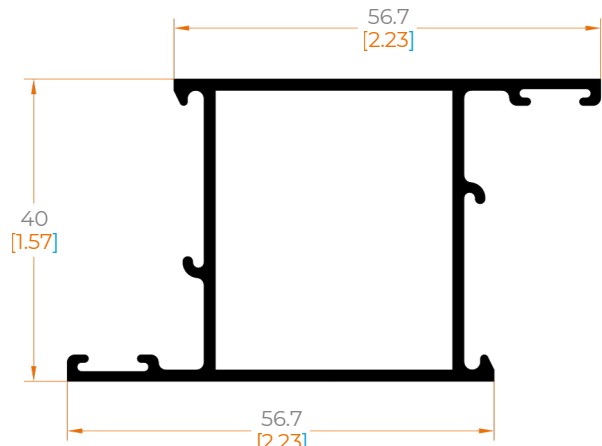
1406 HOJA LISA PUERTA
