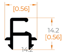
4610 ADAPTADOR MOSQUITERO
