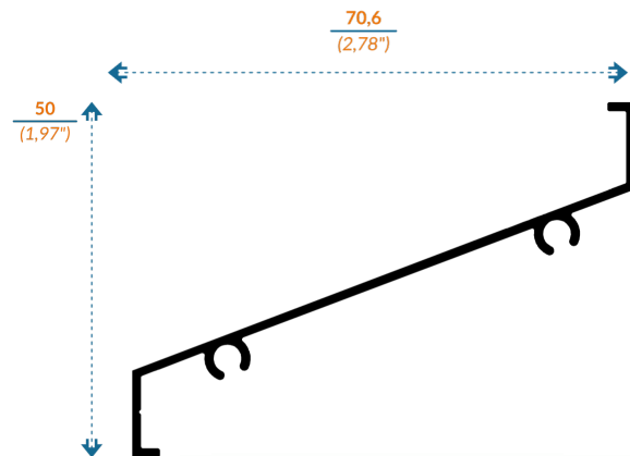
10087 LOUVER 2"
