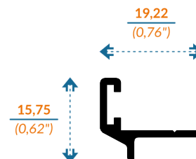
10220/90017 ADAPTADOR OXXO
