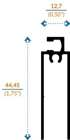
6533 ZOCLO MOSQUITERO
