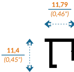
7014/6006 JUNQUILLO
