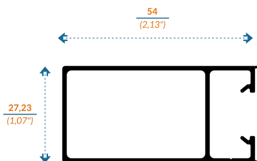
9236 CERCO CHAPA 5.5
