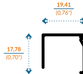
V9088 JUNQUILLO
