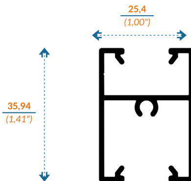
V9082 INTERMEDIO
