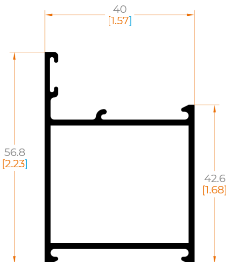
1407 MARCO LISO PUERTA
