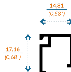
6370 JUNQUILLO
