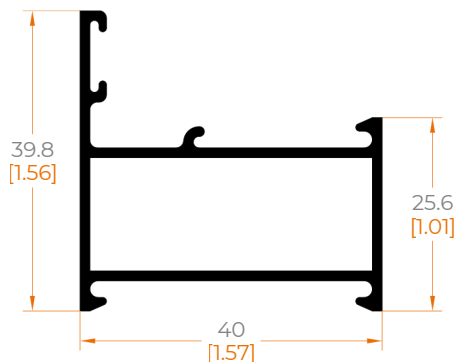
1402 MARCO LISO VENTANA
