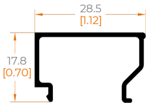
1430 JUNQUILLO ANCHO
