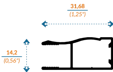
V11035 MARCO ECONÓMICO CERRADO
