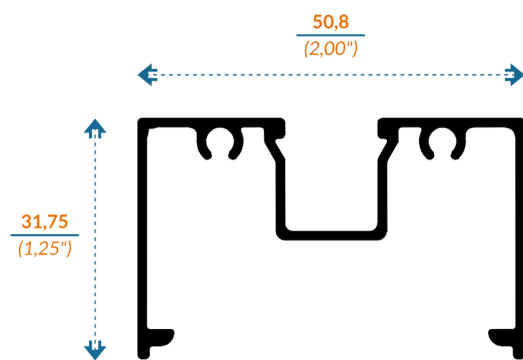
V9083 BOLSA
