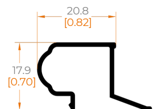
1436 JUNQUILLO RELIEVE ESTRECHO
