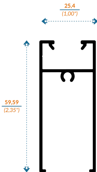
7842 ZOCLO VENTANA
