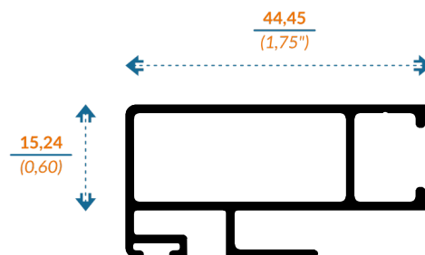
V9955 TRASLAPE PUERTA
