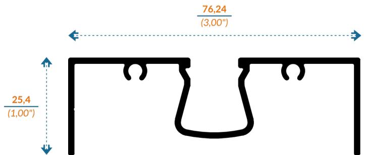
10235 BOLSA CORTA
