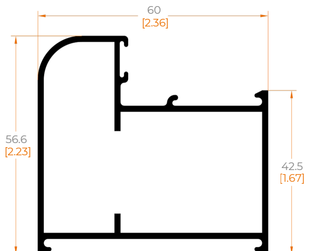
1408 MARCO CURVO PUERTA
