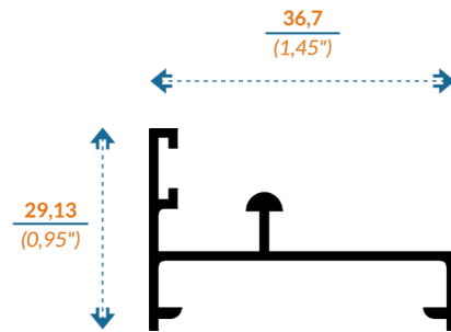
8051 RIEL
