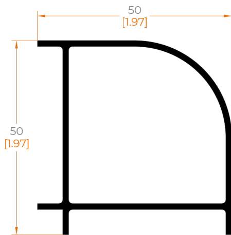
1427 ESQUINERO REDONDO
