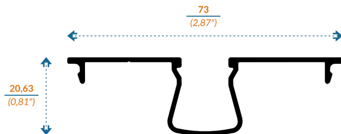
V7315 TAPA BOLSA
