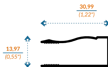
9525/7625 MARCO ECONÓMICO
