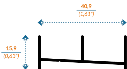
V10198 RIEL INFERIOR LUJO
