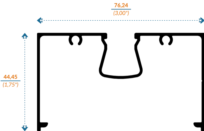
V9135 BOLSA
