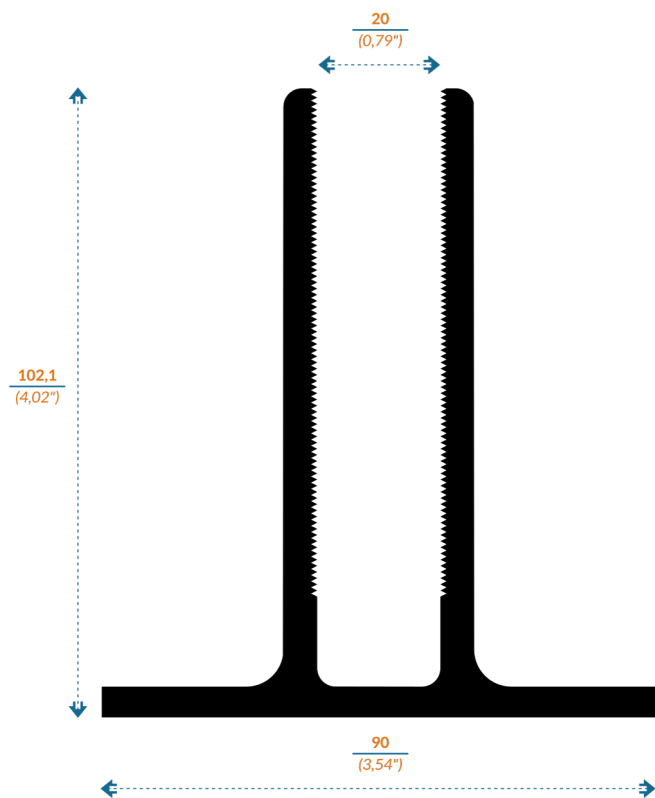
20293 ZOCLO PASAMANOS
