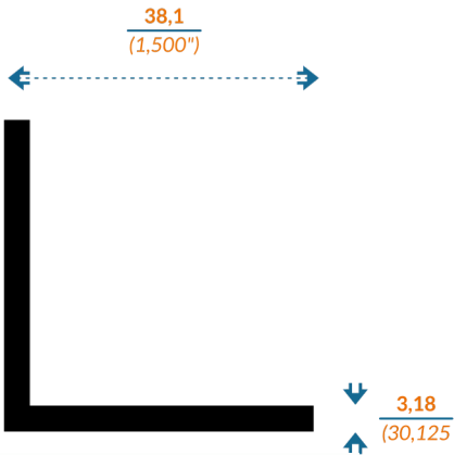
1311 ANGULO 1 1/2 X 1/8"
