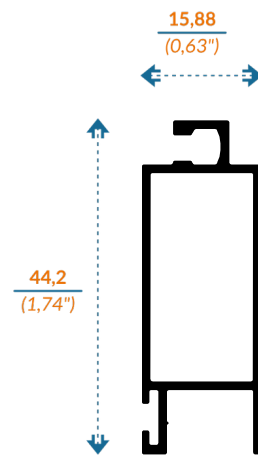
6534 CERCO MOSQUITERO
