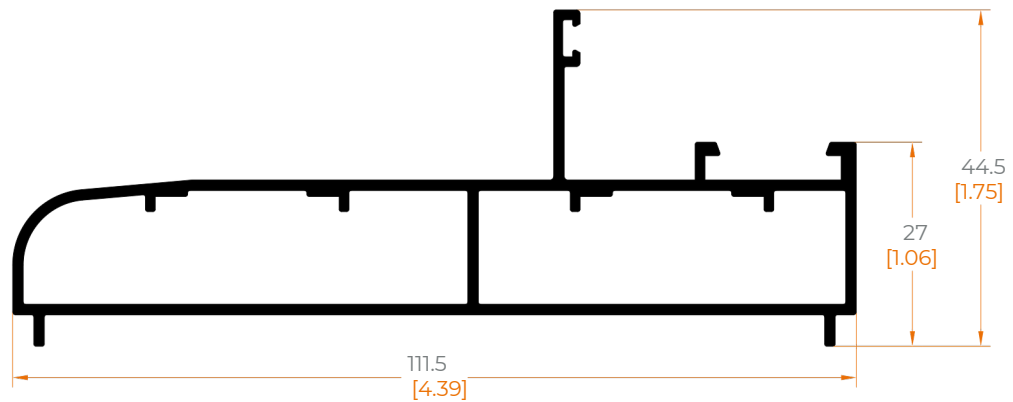
4613 FIJO TUBULAR TRES RIELES
