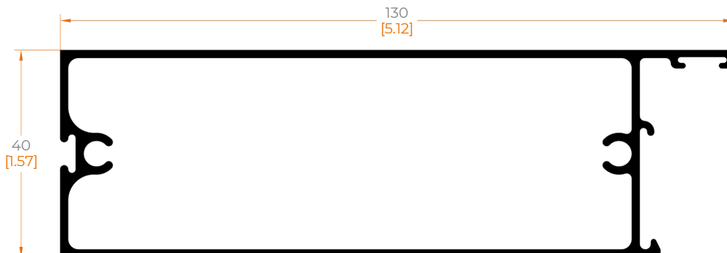
1434 ZOCLO INFERIOR
