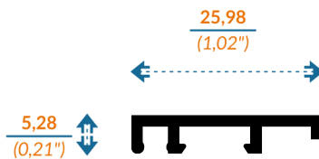
5173/6015 MOSQUITERO PESADO
