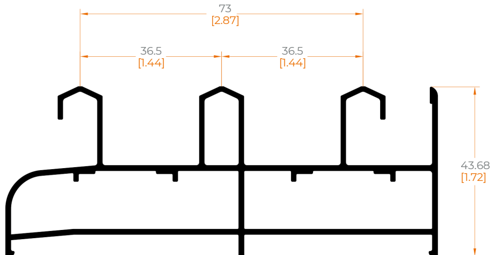
74632 MARCO PERIMETRAL TRES RIELES RECTO
