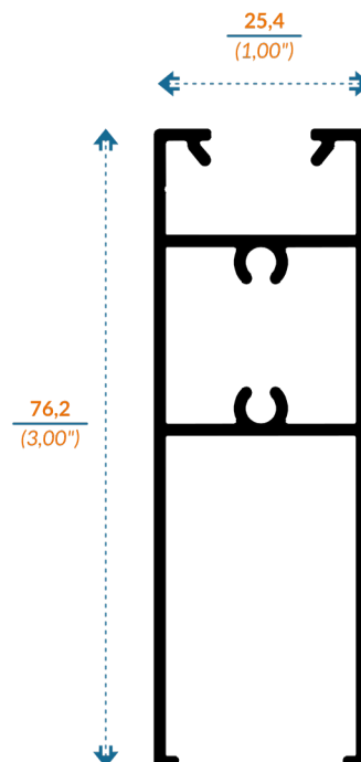
V7842 ZOCLO PUERTA
