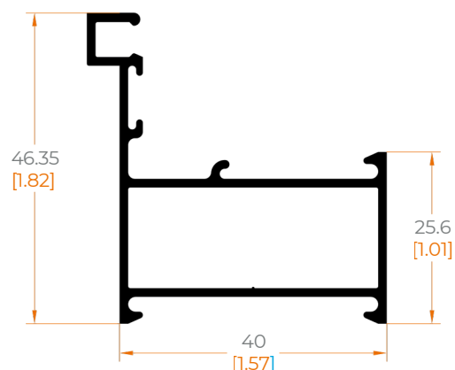
61449 ARRASTRE CON MOSQUITERO
