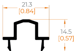
4609 UNION CUATRO HOJAS
