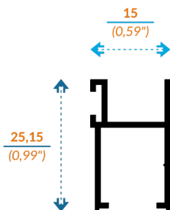
8052 CERCO TRASLAPE
