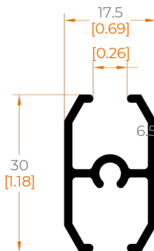
2416 CUADRICULA
