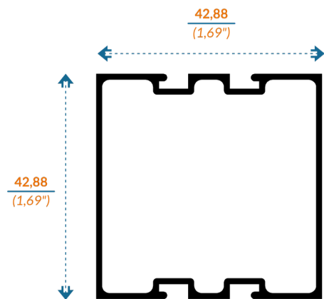
9183/15320 INTERMEDIO
