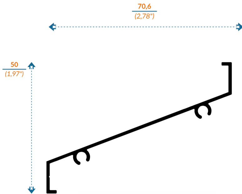
6053 LOUVER 3"
