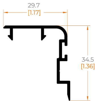
4604 HOJA CENTRAL
