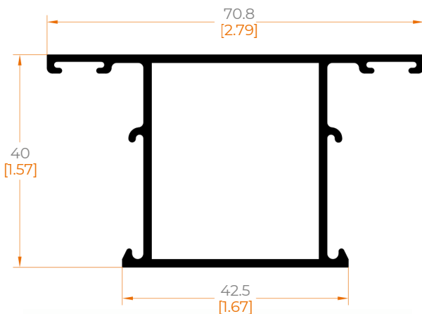
1405 PILASTRA LISA PUERTA
