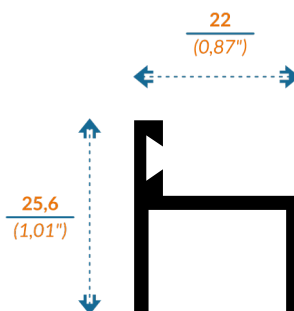
7102/7610 BATIENTE
