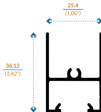
V7836 CABEZAL
