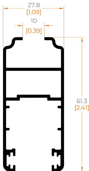
4605 HOJA PERIMETRAL
