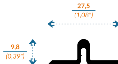
7818/6403 ADAPTADOR
