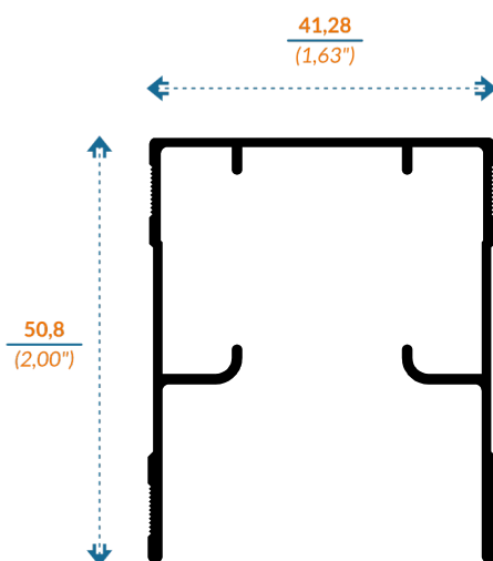
11174/7608 RIEL SUPERIOR
