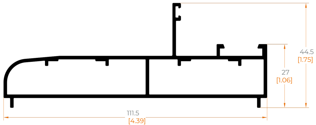
4613 FIJO TUBULAR TRES RIELES
