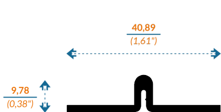
7828/6803 ADAPTADOR
