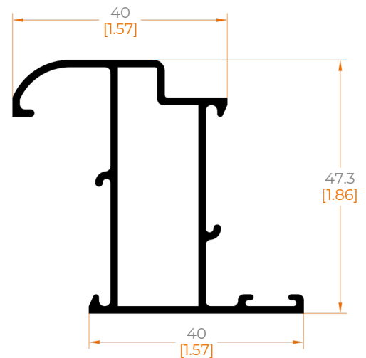
1403 HOJA CURVA VENTANA
