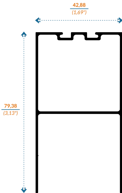
9187/2-5021 ZOCLO
