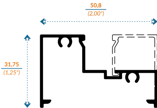
V9084 ESCALONADO
