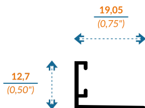
11032/20263 BATIENTE
