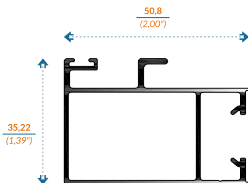
V7848 TRASLAPE PUERTA
