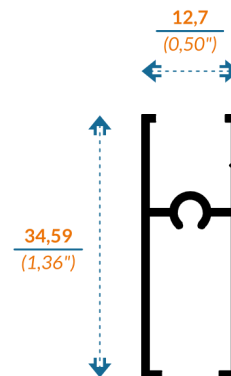
22015 ZOCLO CABEZAL
