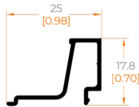
61448 JUNQUILLO 24 MM
