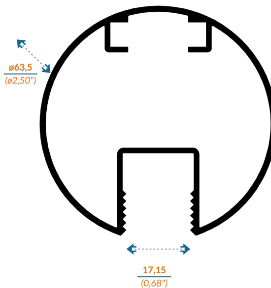
20070 PASAMANOS 2.5"
