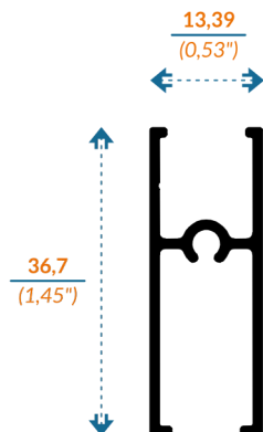
11044 ZOCLO CABEZAL
