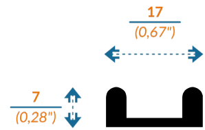
3316/4131 RIEL
