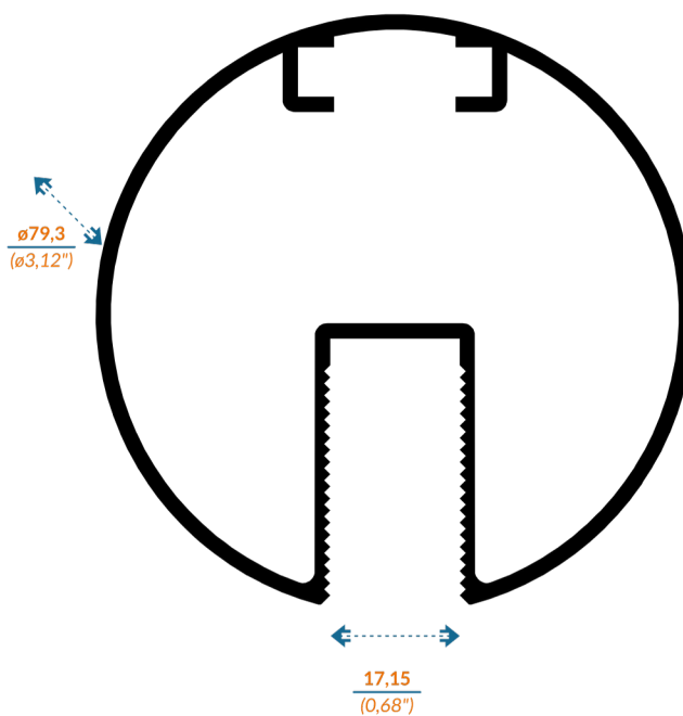
5388 PASAMANOS 3"
