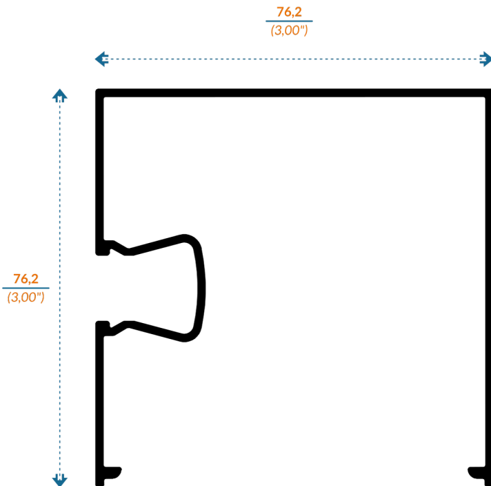
V9115 ESQUINERO
