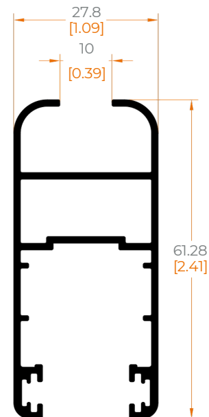
64628 HOJA PERIMETRAL LISA
