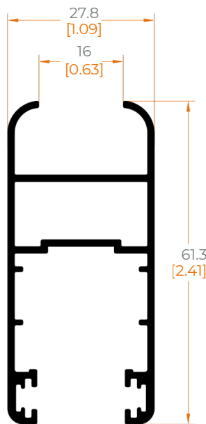
4615 HOJA PERIMETRAL PLAYA
