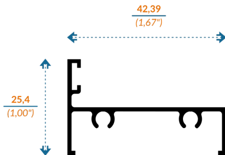
8550 BATIENTE CON VENAS
