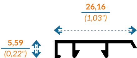
7333 SOLERA MOSQUITERO LIGERO
