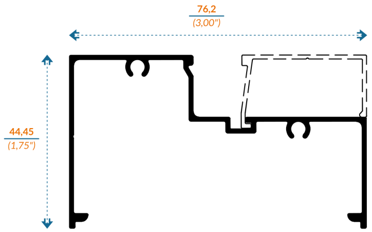
V9136 ESCALONADO
