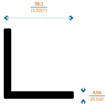
1314 ANGULO 1 1/2 X 3/16"
