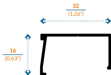
V9112 JUNQUILLO
