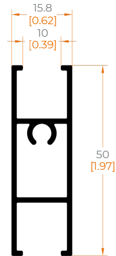
4607 INTERMEDIO
