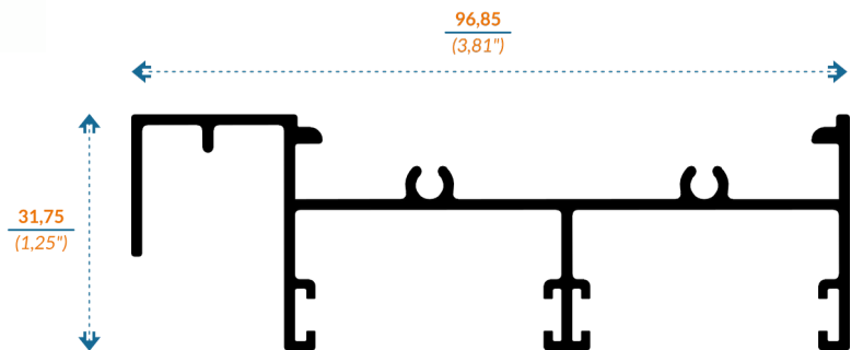
V7862 CHAMBRANA CON MOSQUITERO
