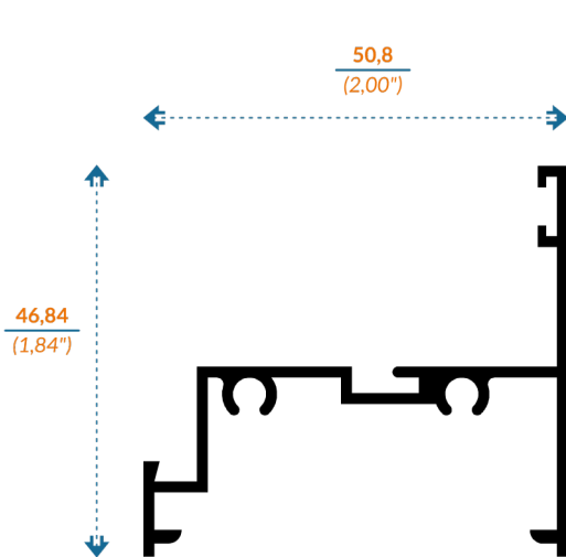
8937/16212 CONTRA MARCO
