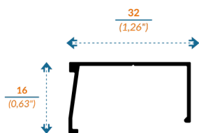
V9112 JUNQUILLO
