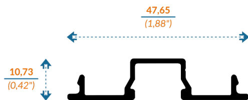
V9085 TAPA BOLSA
