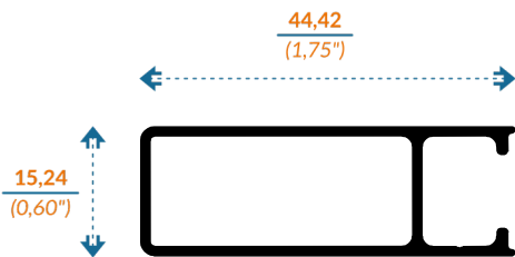
V7821 CERCO PUERTA
