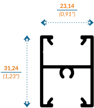
V9081 INTERMEDIO CORTO
