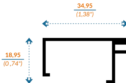
8939 JUNQUILLO VENTILA
