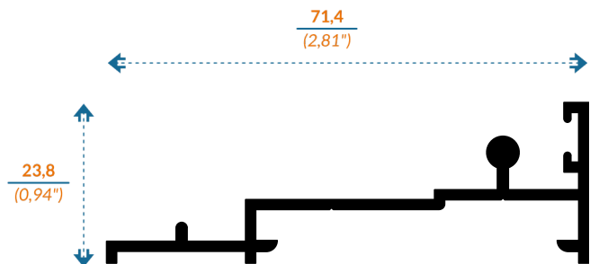
8370/16612 RIEL MOSQUITERO
