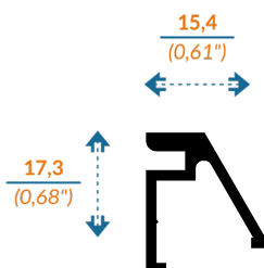
6371/5311 JUNQUILLO BISELADO
