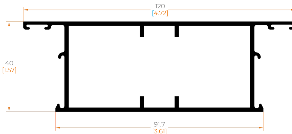
1423 HOJA MONUMENTAL EXTERIOR
