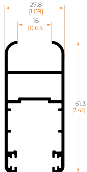
4615 HOJA PERIMETRAL PLAYA
