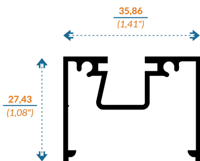
6028 BOLSA
