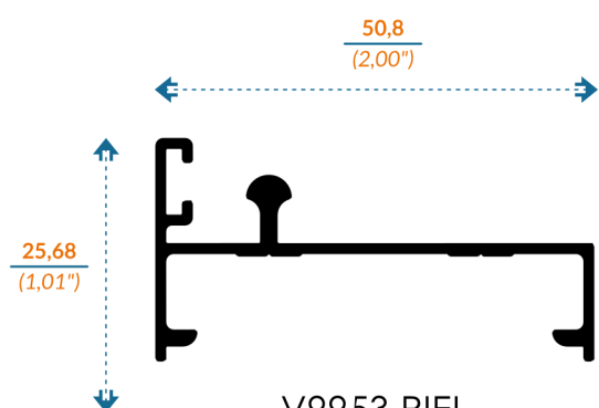
V9953 RIEL
