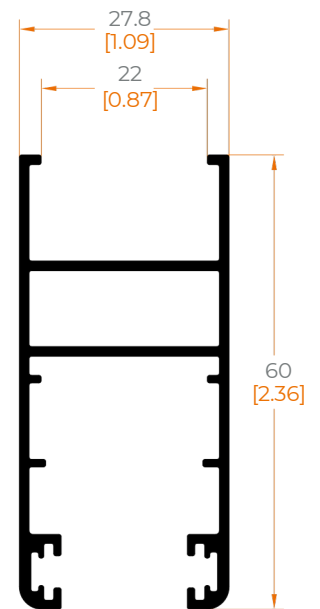
4606 HOJA PERIMETRAL DOBLE VIDRIO
