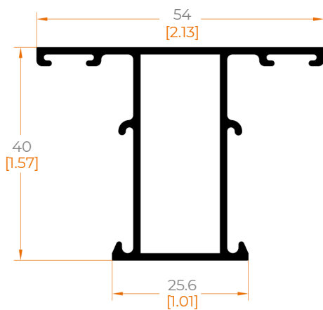
1400 PILASTRA LISA VENTANA
