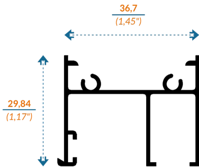
8050 CHAMBRANA
