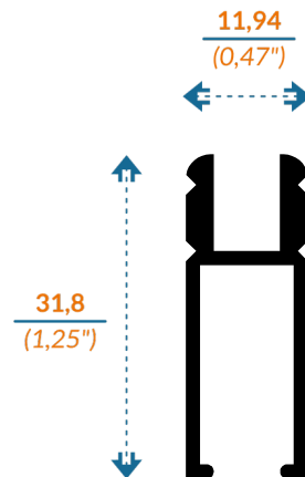
3358/4132 ZAPATA
