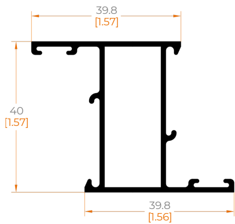
1401 HOJA LISA VENTANA
