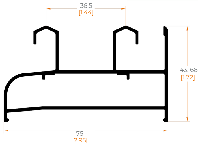
4610 ADAPTADOR MOSQUITERO
