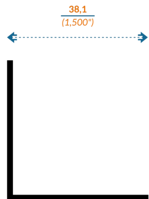
1320 ANGULO 1 1/2" x 1/16
