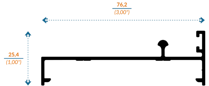
9957/17016 RIEL
