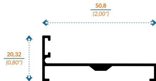
5844 BATIENTE SIN VENAS
