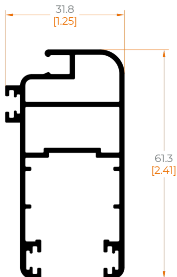
64624 HOJA PERIMETRAL MOSQUITERO
